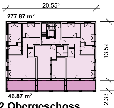
2.Obergeschoss
