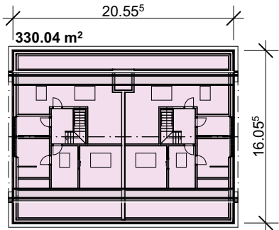
Dachgeschoss
