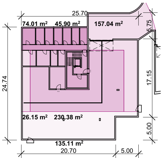
Untergeschoss
