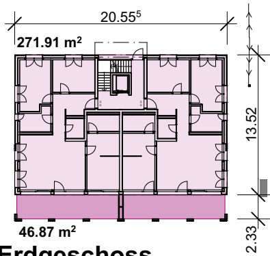
Erdgeschoss
