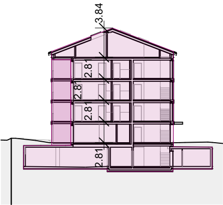
Schnitt A-A
