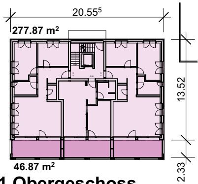
1.Obergeschoss
