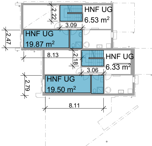
Untergeschoss - Bestand
