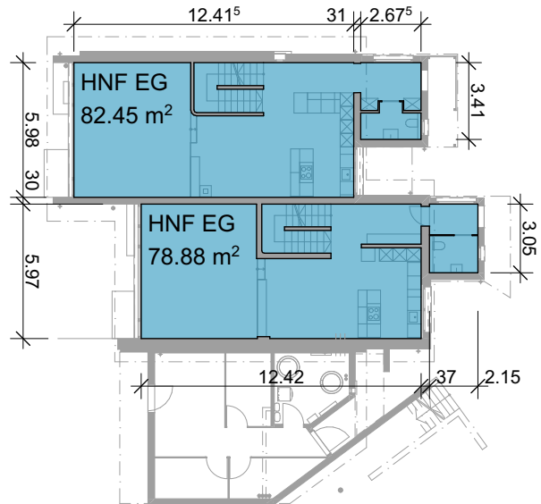
Erdgeschoss - Bestand
