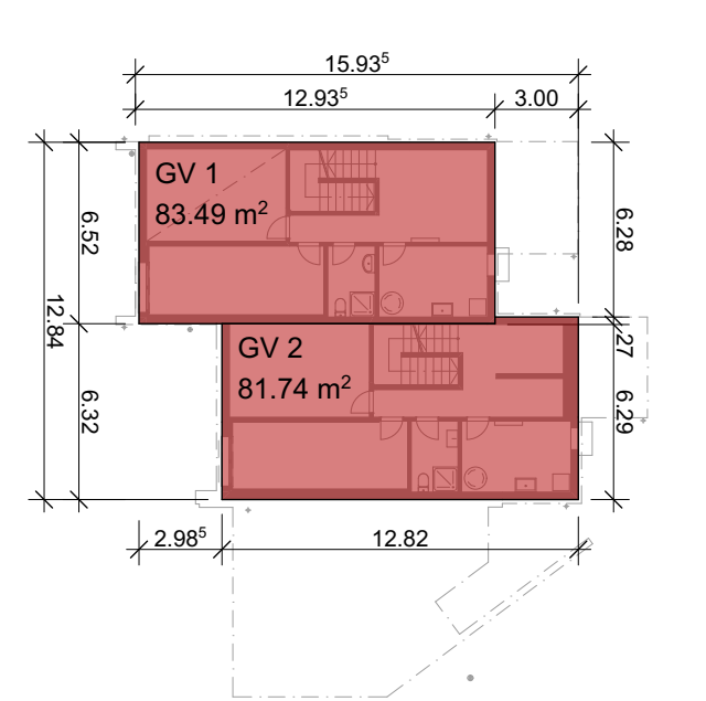
Untergeschoss - Bestand
