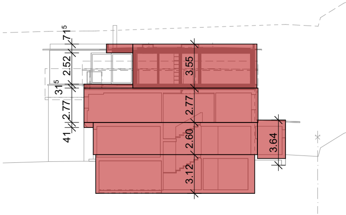
Schnitt B
