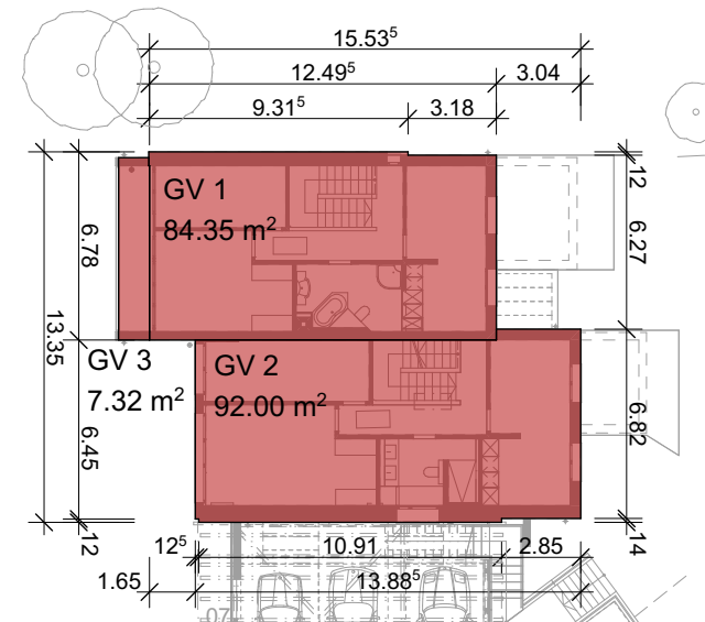
1. Obergeschoss - Bestand
