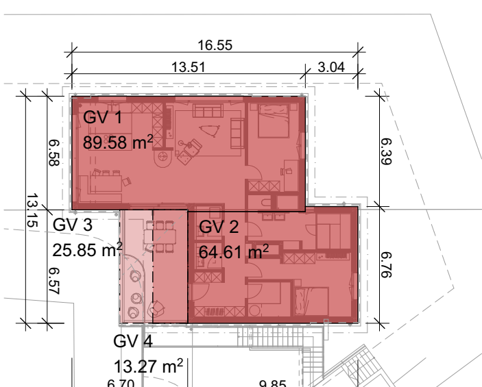
2. Obergeschoss - Neubau
