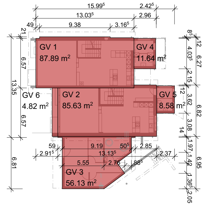
Erdgeschoss - Bestand
