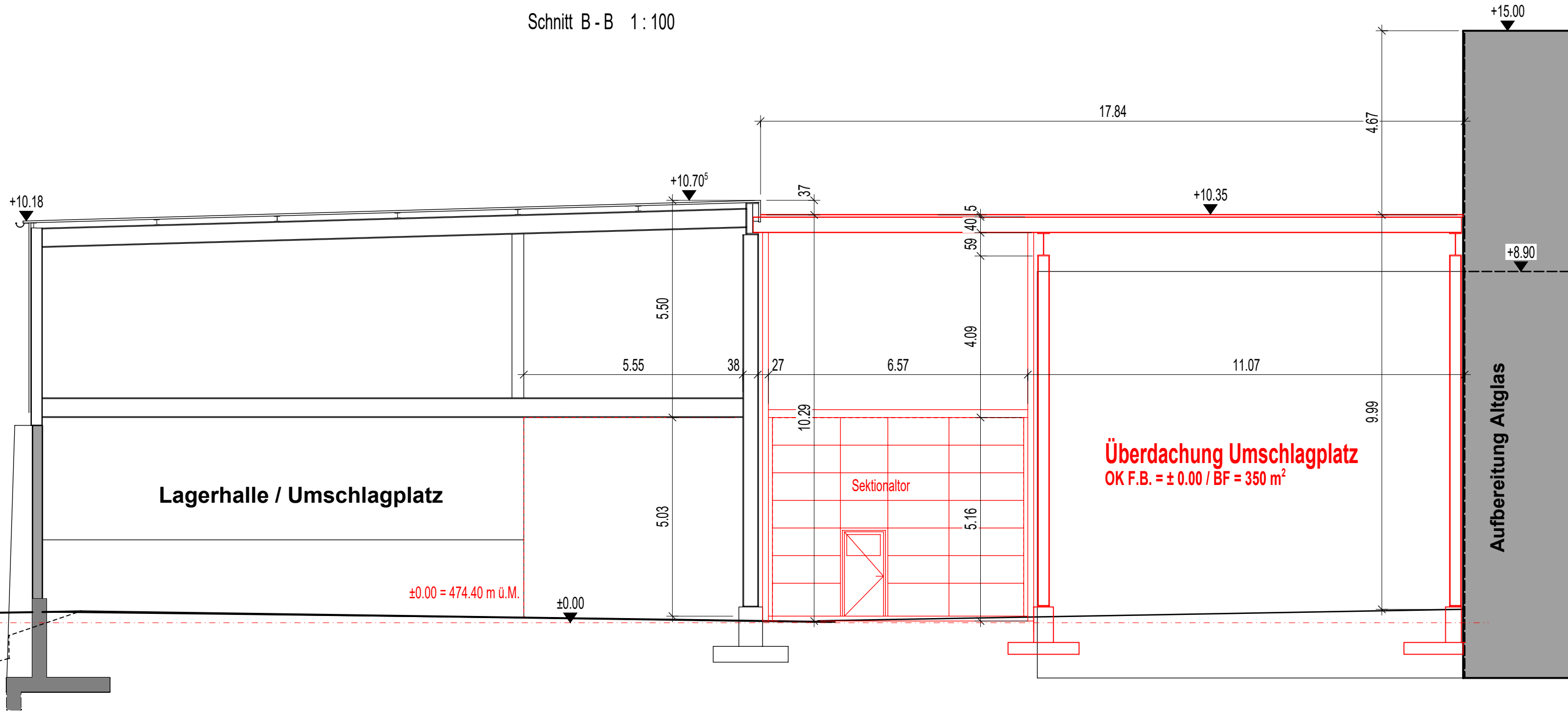
Schnitt B - B 1:100
