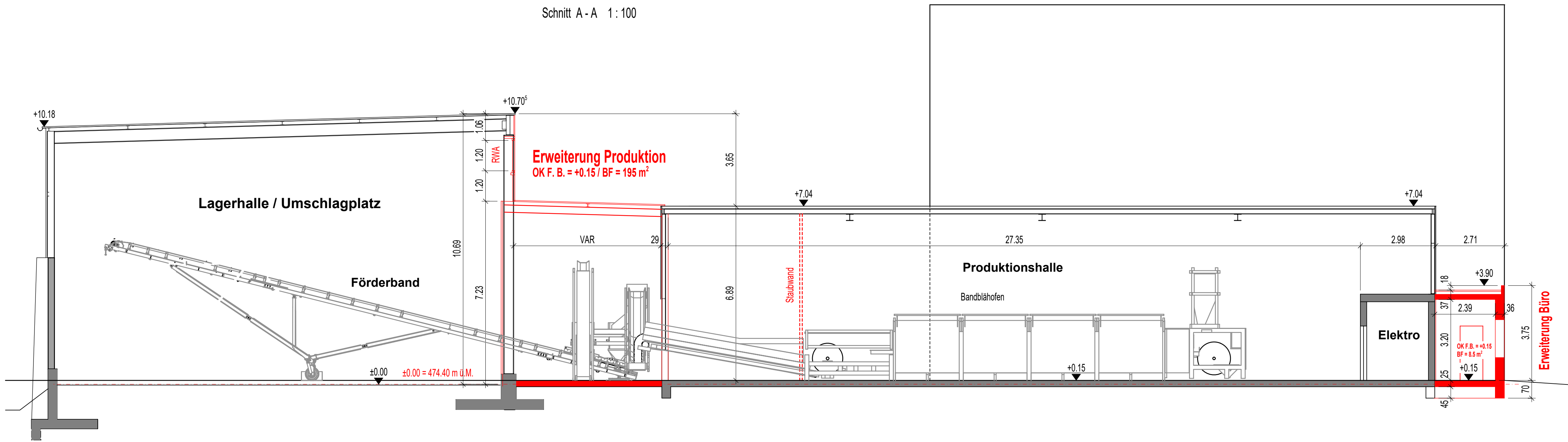
Schnitt A - A 1:100
